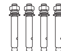
固定用アンカー (M10x115mm)×4
